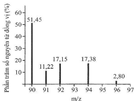
Phổ khối lượng của zirconium
