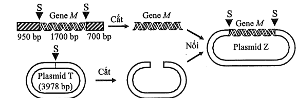
Ghi chú: ▼ là vị trí nhận biết của enzyme giới hạn S; các số thể hiện kích thước của các đoạn DNA hoặc plasmid (bp: cặp nucleotide)
