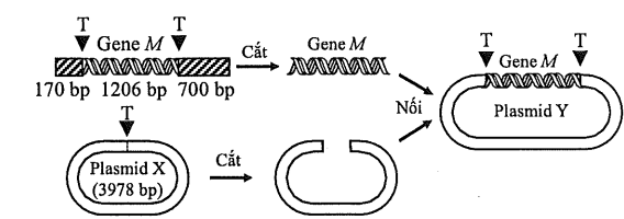
Ghi chú: ▼ là vị trí nhận biết của enzyme giới hạn T; các số thể hiện kích thước của các đoạn DNA hoặc plasmid (bp: cặp nucleotide)
