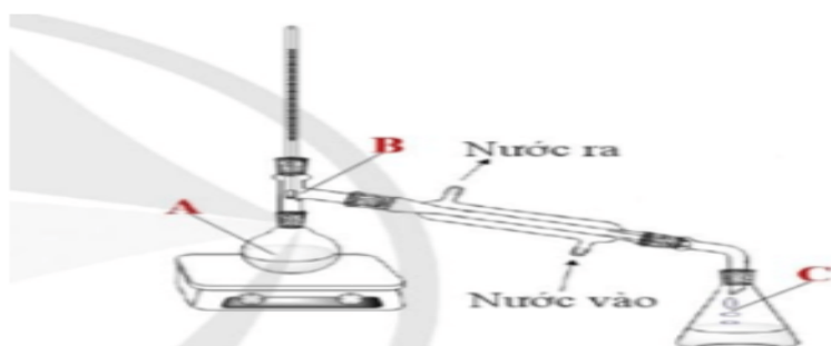
Hình 9.5. Dụng cụ tách các chất lỏng ra khỏi nhau
