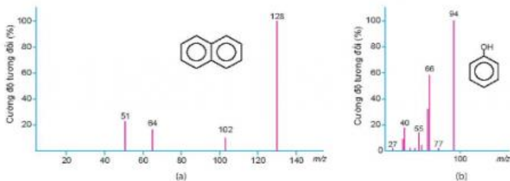
▲ Hình 10.1. Phổ khối lượng của naphthalene (a) và phenol (b) (1)
