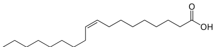
Oleic acid (nhiệt độ nóng chảy 14^\circ C )
