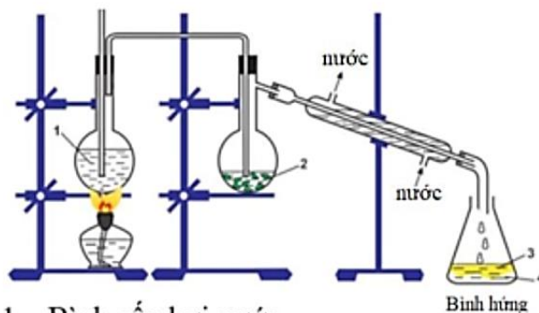
1. Bình cấp hơi nước. 2. Bình chứa nguyên liệu chưng cất.
