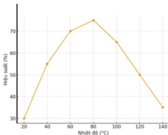
Ảnh hưởng của nhiệt độ đến hiệu suất tổng hợp ethyl acetate
